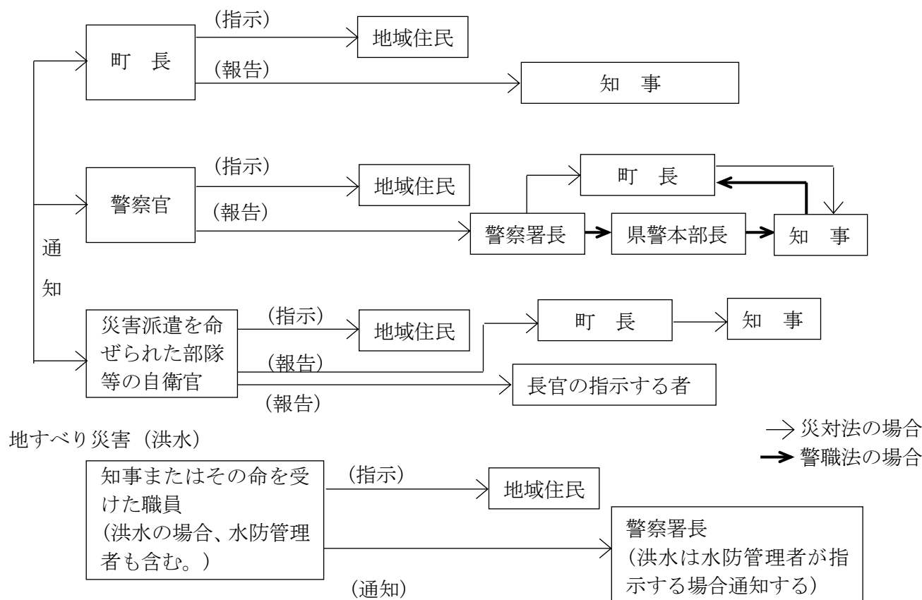
〔避難指示系統図〕
